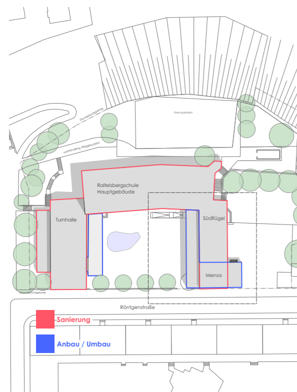
Lageplan
